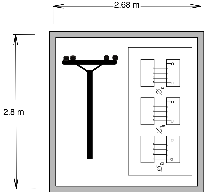
SUBESTACIÓN ELÉCTRICA
